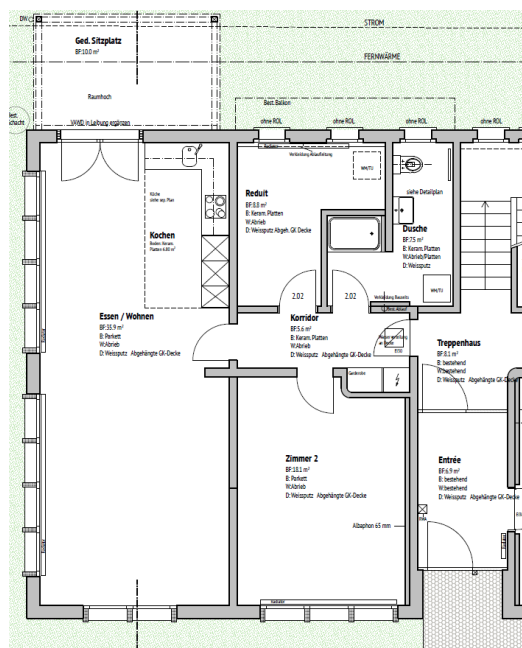
Grundriss Wohnung Erdgeschoss
