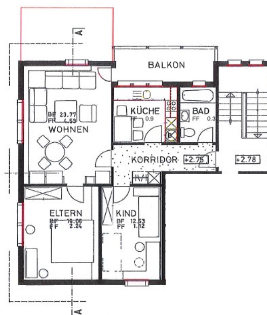
Grundriss Wohnung 1. Stock
