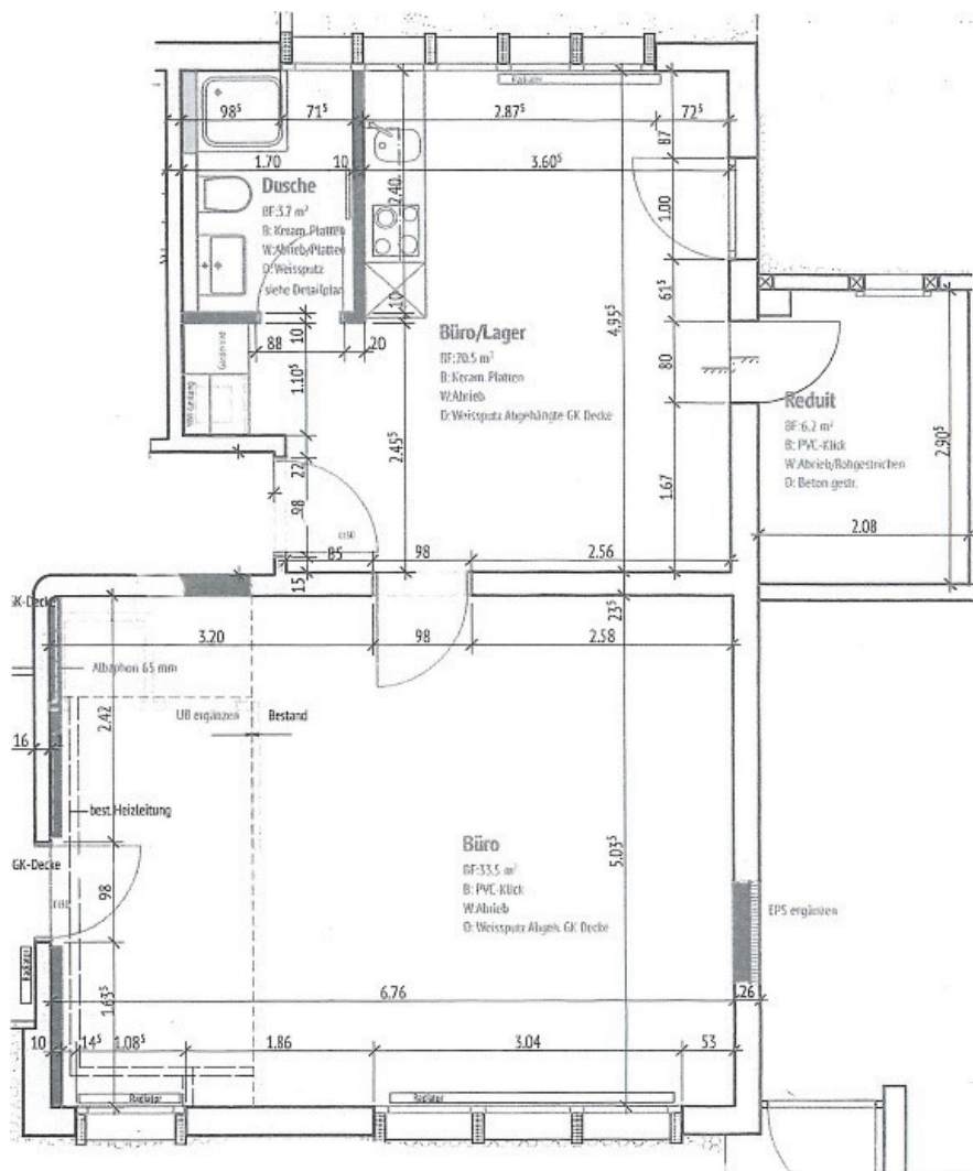
Grundriss 1.5-Zimmer-Wohnung/ Büro oder Therapieraum
